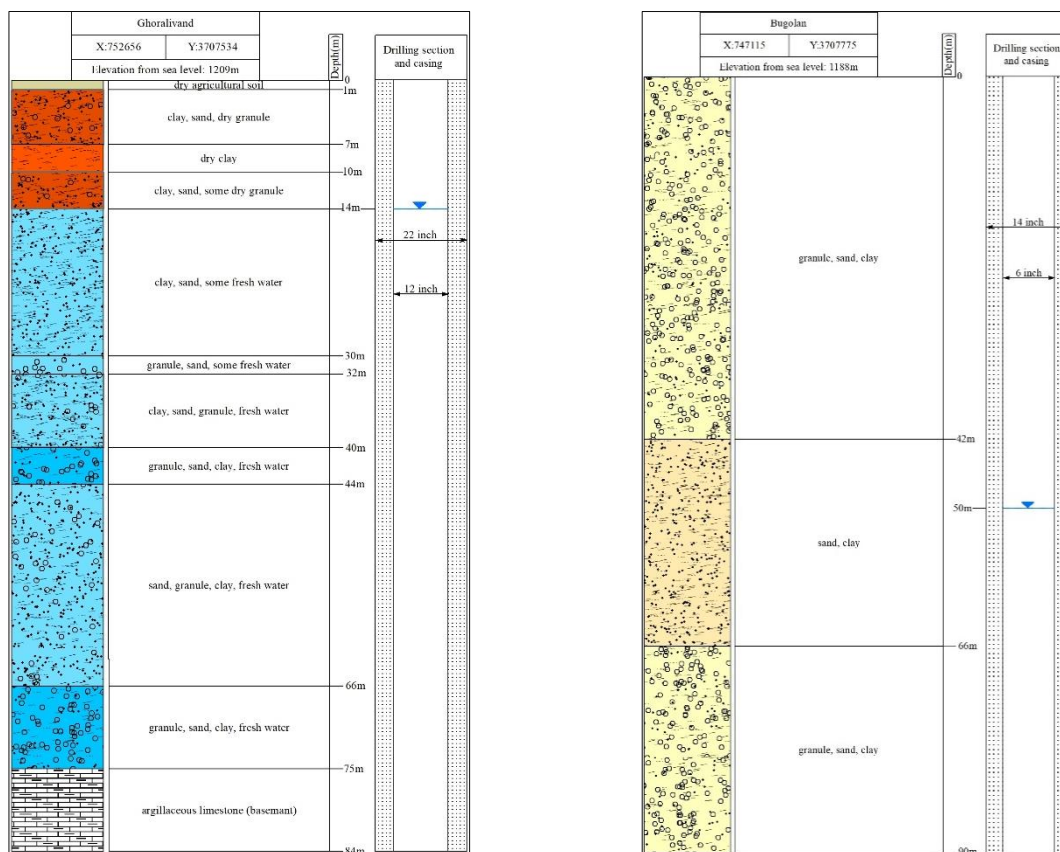
شکل ۶. نمونه لاگ چاه‌های اکتشافی دشت کوهدشت، لاگ چاه بوگلان (سمت راست) و لاگ چاه قرعلیوند (سمت چپ)
