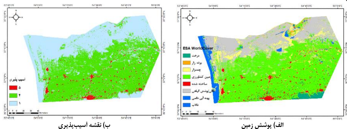
شکل ۷. پوشش زمین و نقشه آسیب‌پذیری منطقه آق‌قلا
