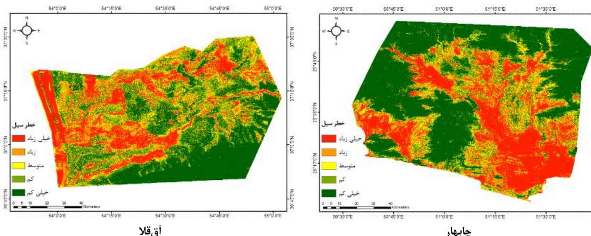
شکل ۵. نقشه خطر سیل بازطبقه‌بندی‌شده در مناطق چابهار و آق‌قلا
