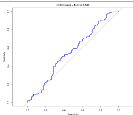
شکل ۵. نمودار ROC ریسک زمین‌لغزش شهرستان قزوین با استفاده از مدل رگرسیون لجستیک
